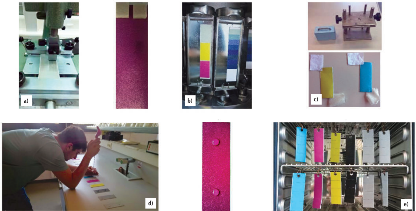
Slika 2. Ispitivanje postojanosti otiska na: a) suho i mokro trljanje, b) djelovanje umjetnog svjetla, c) djelovanje vode, d) vodene kapi, e) ubrzano starenje djelovanjem topline
